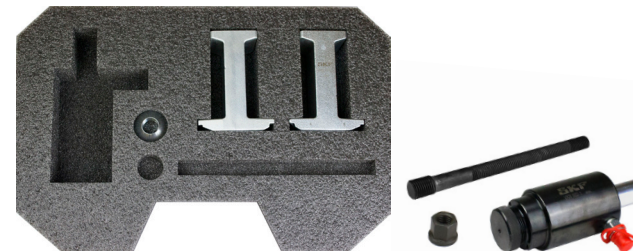
VKN 601: herramienta de desmontaje de rodamientos HBU 2.1. La caja cuenta con un espacio reservado especialmente para complementar el kit con el cilindro hidráulico opcional VKN 602-1.
